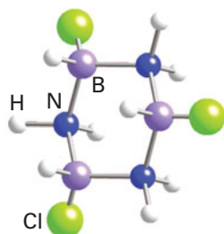
25 B_3N_3H_3Cl_3
