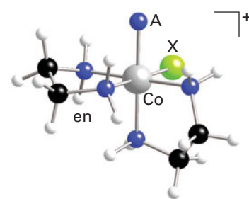
8 cis -[CoAX(en) 2 ] +
