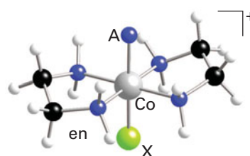
9 trans -[CoAX(en) 2 ] +
