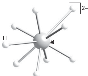
8 [\text{ReH}_9]^{2-}
