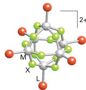
26 [\text{M}_6\text{X}_{12}\text{L}_6]^{2+}
