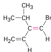
( E )-1-Bromo-2-isopropyl-1,3-butadiene
