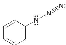
Azidobenzene
