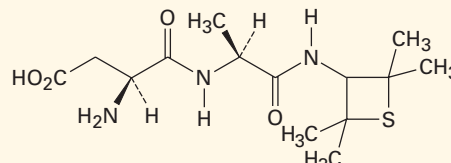
Alitame
