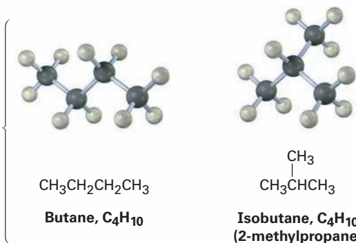
\text{CH}_4 \text{CH}_3\text{CH}_3 \text{CH}_3\text{CH}_2\text{CH}_3 Methane, \text{CH}_4 Ethane, \text{C}_2\text{H}_6 Propane, \text{C}_3\text{H}_8
