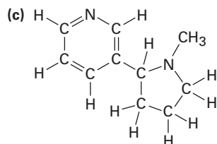
Nicotine
