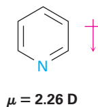
\mu = 2.26 D
