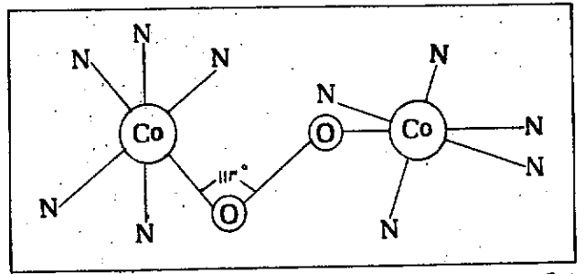
شکل ۱- فرمول ساختمانی \mu - پروکسوئیس [پنتا آمین کبالت (III)] در این نمودار اتمهای هیدروژن حذف شده‌اند.
