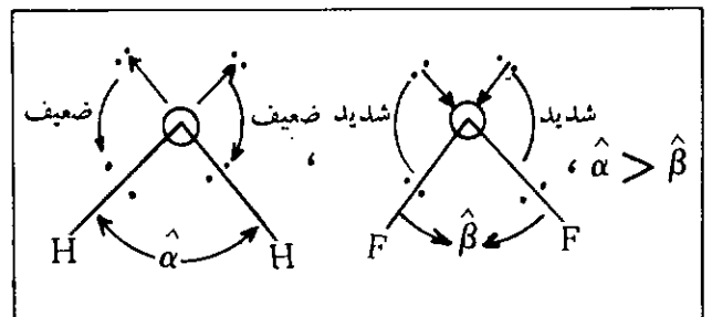
شکل ۵- مقایسه تأثیر دافعه الکترونها غیر پیوندی اتم مرکزی در مولکولهای H_2O و OF_2
