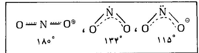
شکل ۱- ساختار مولکولی NO_2^+ ، NO_2 و NO_2^- و مقایسه زاویه پیوندی آنها
