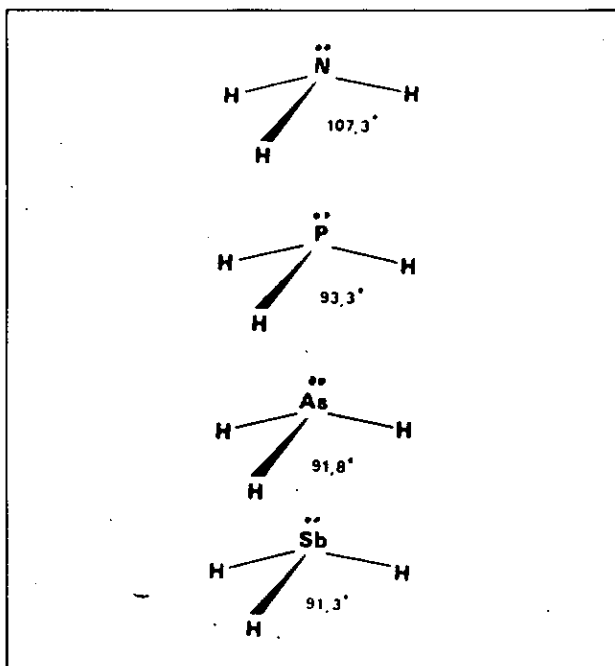
شکل ۹- روند تغییر زاویه پیوندی در مولکولهای هرم مثلثی XH_3 :
