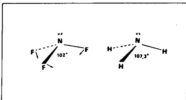
شکل ۱۱- مقایسه اندازه زاویه پیوندی در مولکولهای NF_3 و NH_3
