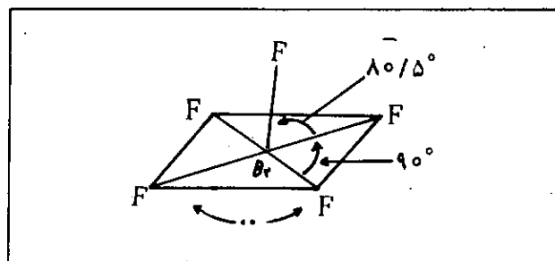
شکل ۳- وضعیت زوایای پیوندی در مولکول BrF_5
