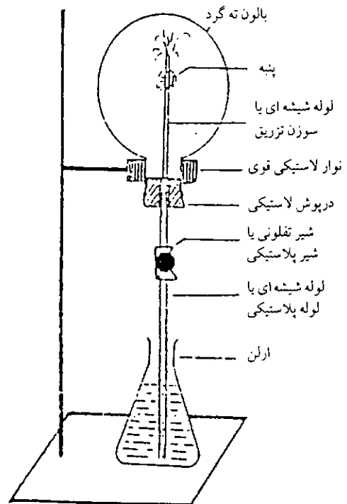
شکل ۱ وضعیت دستگاه به هنگام تعیین درصد اکسیژن هوا
