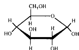
گلوکز - D - α
