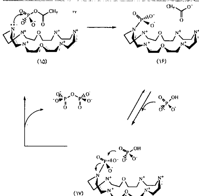
شکل ۲ ستر پیروفسفات CH_3CO_2PO_3^{2-} = ACP = استیل فسفات
